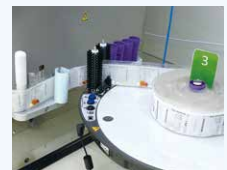
「パーソナルワン」の全自動錠剤分包機
